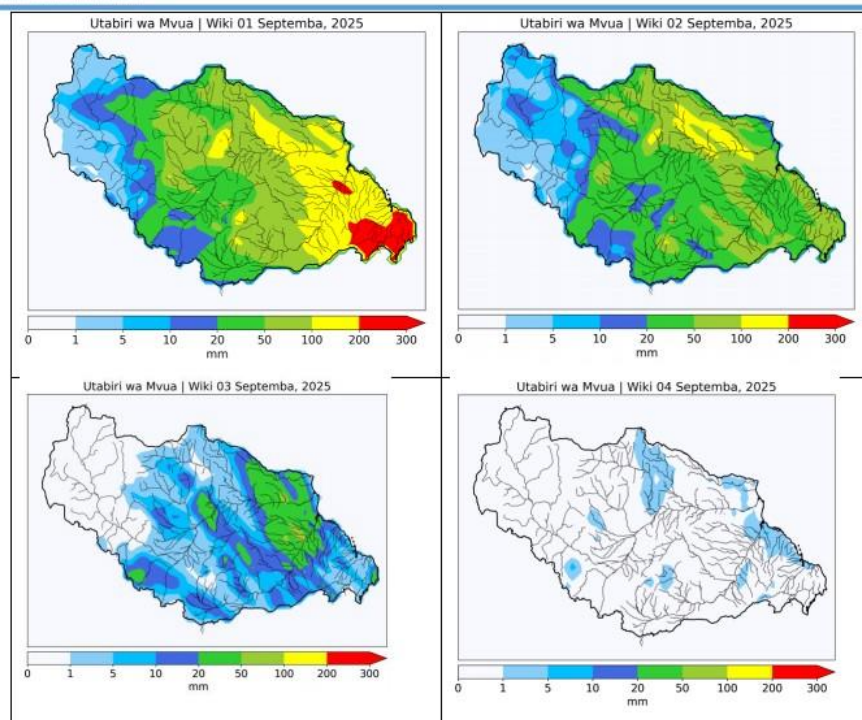
Kielelezo 1: Utabiri wa mvua kwa kipindi cha kila wiki ya mwezi Septemba 2025 katika eneo la bonde la Wami/Ruvu
