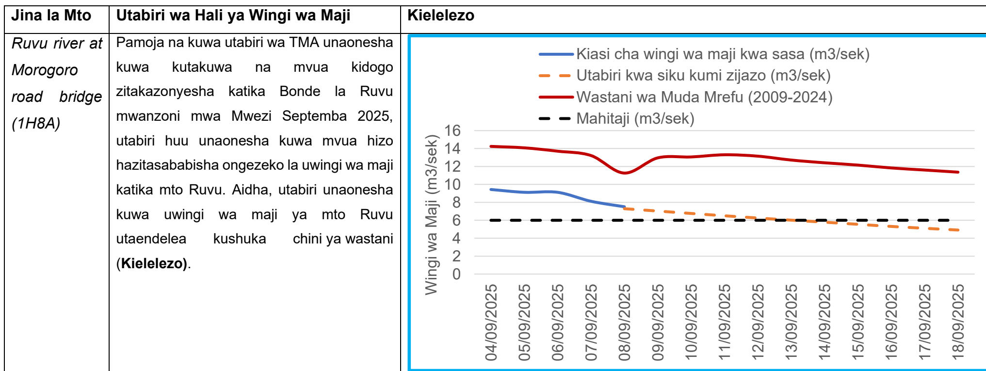
Jendwali Na. 1: Utabiri wa hali ya wingi wa maji Mto Ruvu katika kituo cha Ruvu river at Morogoro road bridge (1H8A) .
